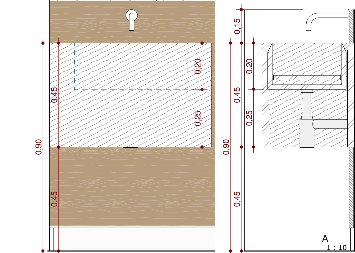
01- DET. BANCADA 1 : 10
